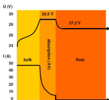
Krzywa ładowania
